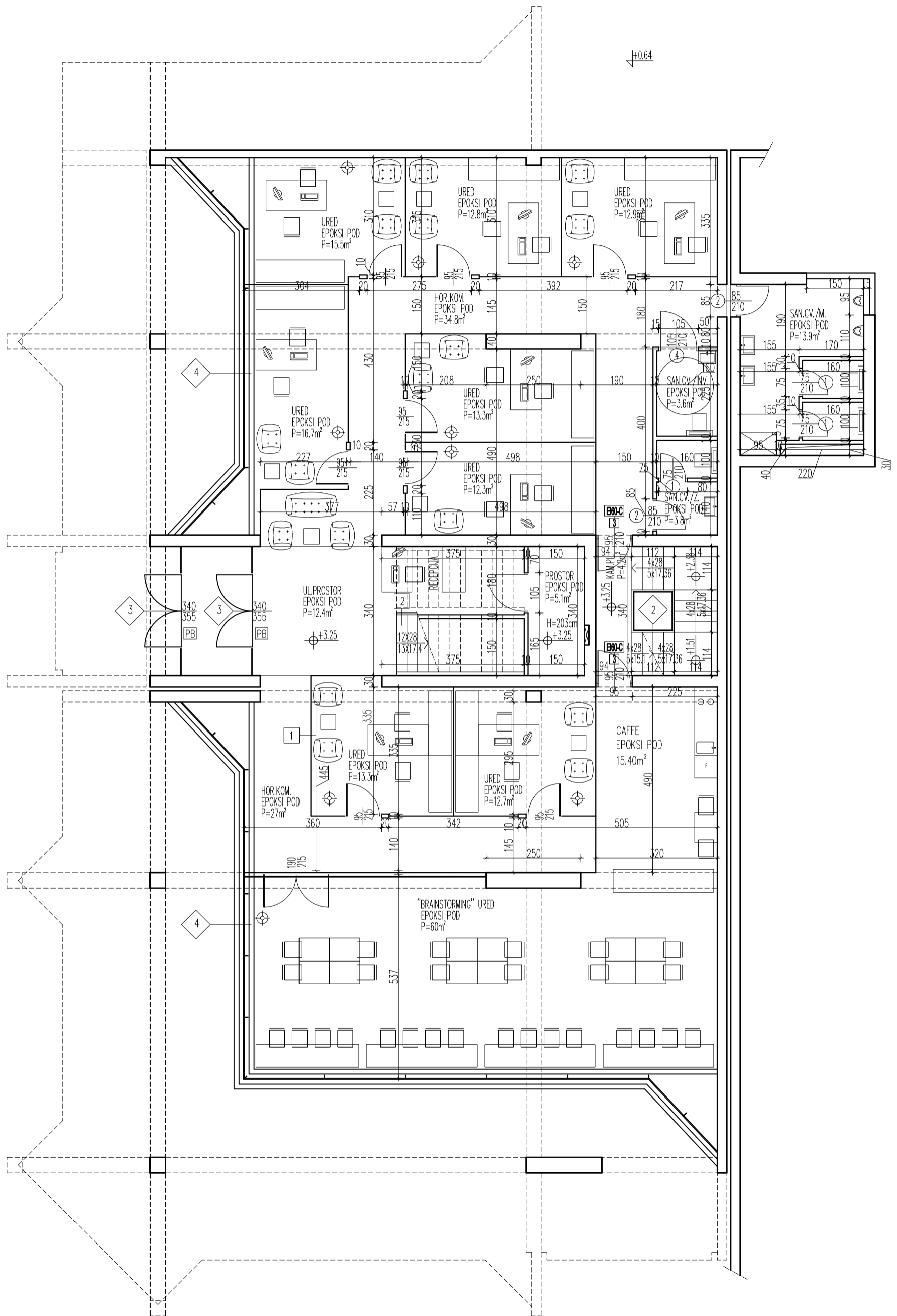
TLOCRT PRIZEMLJA
